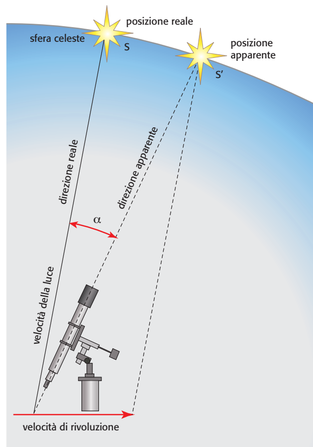
Figura 1 Il fenomeno dell'aberrazione stellare. L'angolo di aberrazione \alpha è l'angolo che si forma tra la direzione vera della stella e la direzione apparente. Quest'ultima è inclinata nel senso della velocità di rivoluzione della Terra.
