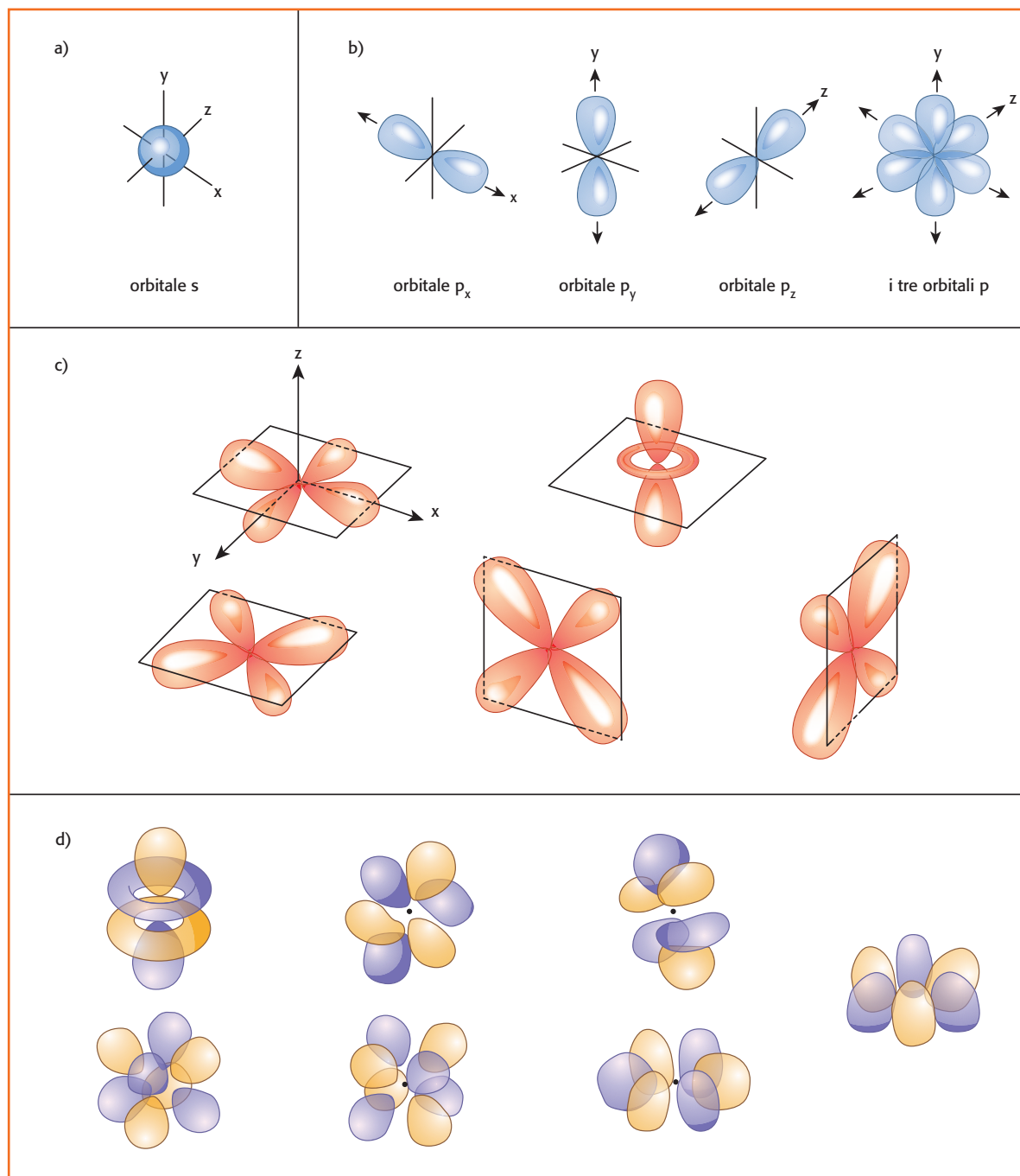
▼ Fig. 1 Le forme dei diversi orbitali: a) orbitale s; b) orbitali p; c) orbitali d; d) orbitali f.
