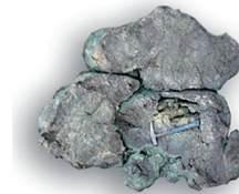
Figura 3 Ofioliti.
