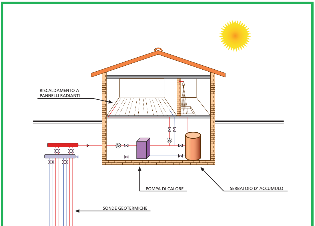
SCHEMA CIRCUITO CHIUSO TERRA/ACQUA (SONDE GEOTERMICHE VERTICALI)
