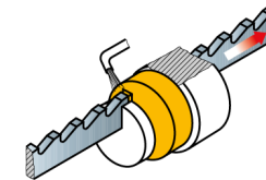
Brocciatura di una cava per linguetta
