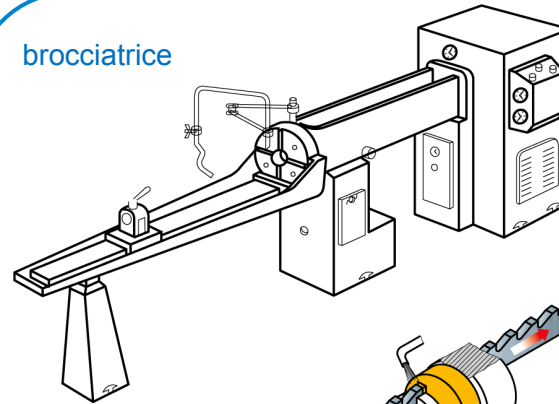
Brocciatura di una cava per linguetta
